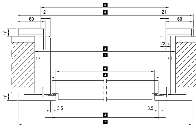
Vízszintes metszetek
