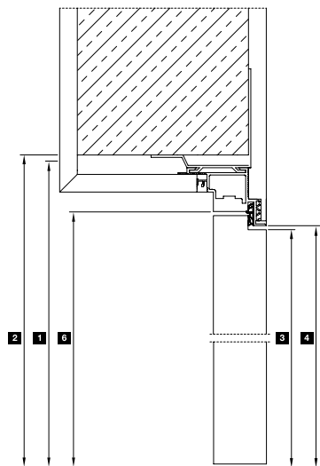
Ellenkezőleg nyíló ajtólap függőleges metszete
