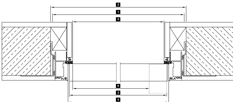
Falcolatlan ajtólap vízszintes metszete
