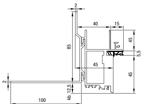
Zeroline ajtók méretezése
