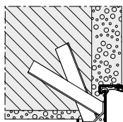
Beépítés horgonyos rögzítőelemmel
