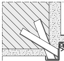
Beépítés horgonyos rögzítőelemmel
