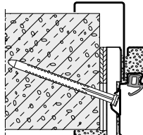
Átlós rögzítés Vario B53 kiegészítőkkel, mint 2-héjű befoglalótok (gázbeton)
