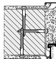
Sarok- és kiegészítőtok Beépítés tiplis rögzítőfülekkel
