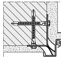
Beépítés tiplis rögzítő- fülekkel
