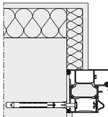
Blokktok Szerelés szerelőnyíláson át
