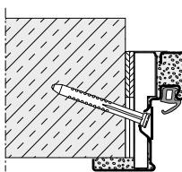
Átlós rögzítés (nem vakolt téglafal / betonfal)
