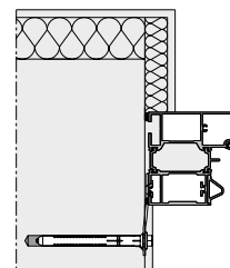
Blokktok Szerelőfüles rögzítés
