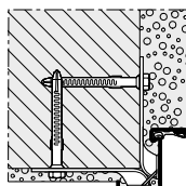
Beépítés tiplis rögzítőfülekkel
