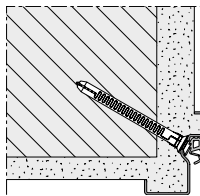
Speciális saroktok Átlós rögzítéssel a falon keresztül
