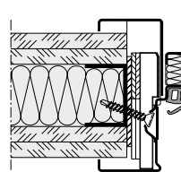
Átlós rögzítés (Gázbeton)
