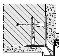
Einbau mit Dübel- anker
