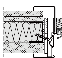
Diagonalbefestigung (Porenbeton)
