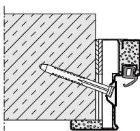
Diagonalbefestigung (Sichtmauerwerk / Beton)
