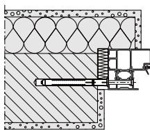
Blockzarge Tütungsmontage
