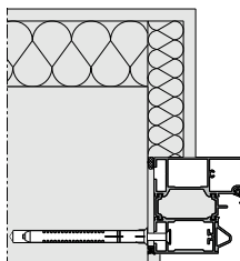
Blockzarge Tütungsmontage
