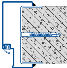
Schweißmontage Porenbeton D Typ 2
