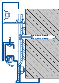
Verdeckte Montage Sichtbeton / Sichtmauerwerk D Typ 3
