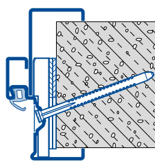
Diagonalbefestigung Porenbeton C Typ 1
