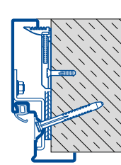
Diagonalbefestigung Sichtbeton / Sichtmauerwerk bis MW 450 D Typ 1
