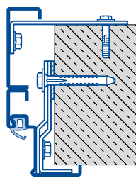
Laibungsmontage Mauerwerk C Typ 3
