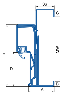
DryFix-Zarge mit Ergänzungszarge Vario B36 bis RC2 B Typ 2
