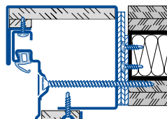
Schraubmontage Montagewand F90A E Typ 2
