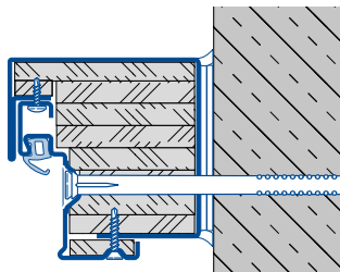
Dübelmontage Mauerwerk E Typ 2
