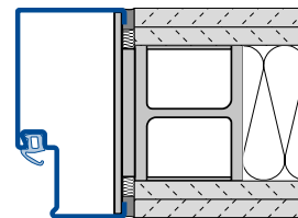
Schweißmontage Stahlkonstruktion E Typ 1
