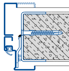
NEU. Schweißmontage Porenbeton C Typ 3
