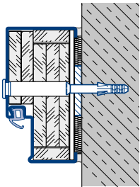
Dübelmontage Mauerwerk, geputzt E Typ 1
