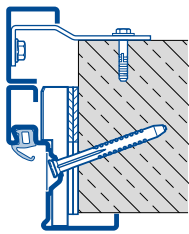
Diagonalbefestigung Mauerwerk C Typ 2
