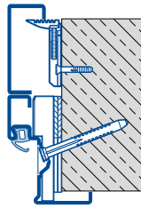
Diagonalbefestigung Sichtmauerwerk / Sichtbeton C Typ 2
