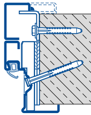
Diagonalbefestigung Sichtmauerwerk / Sichtbeton C Typ 2
