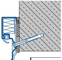
Diagonalbefestigung Mauerwerk / Beton / Porenbeton B Typ 1
