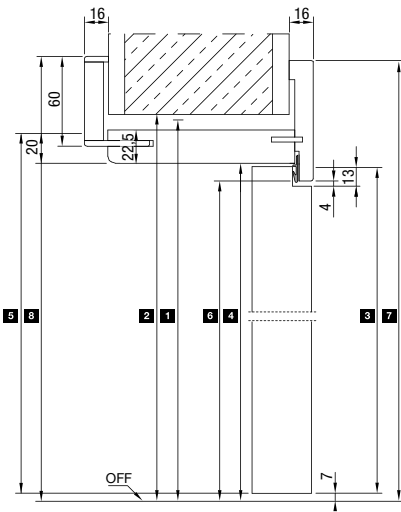
Verticale doorsnede
