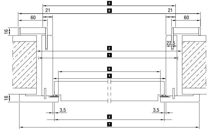
Horizontale doorsneden
